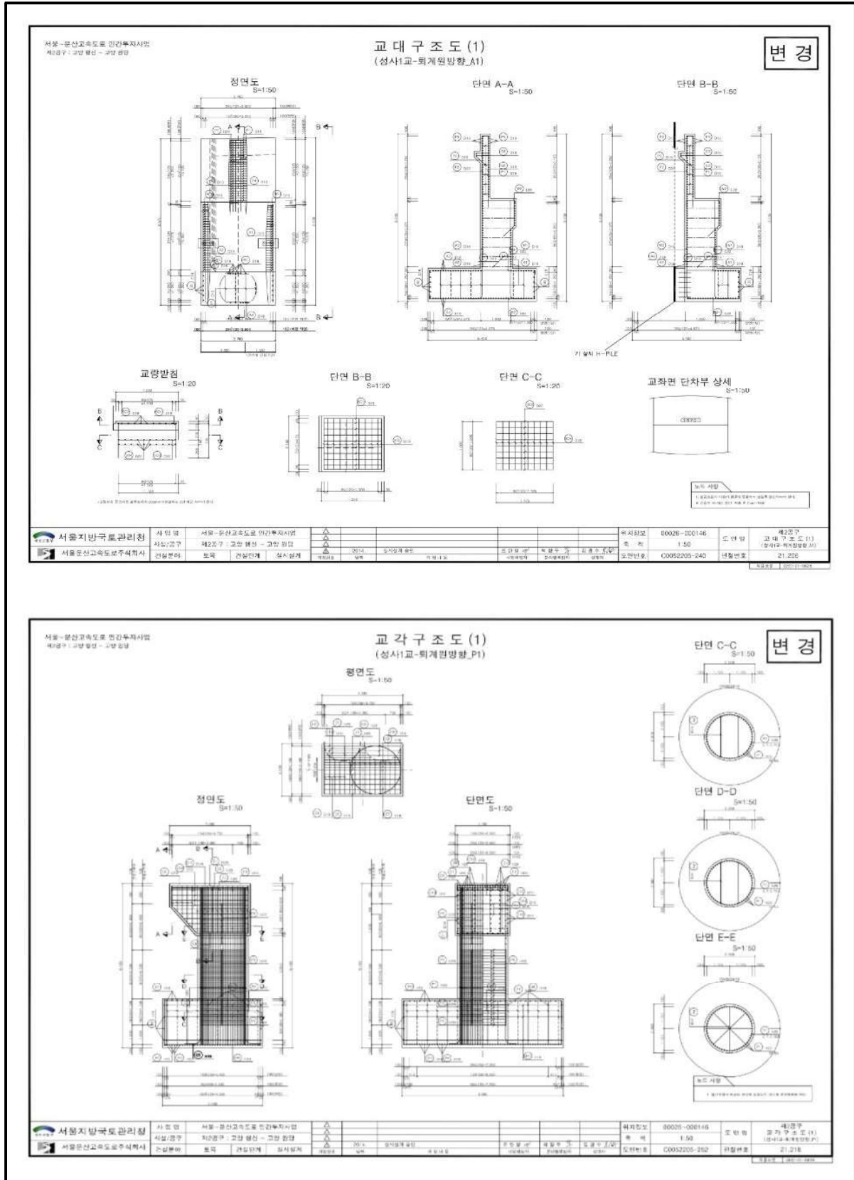
【그림 25.1.7】 교대 및 교각 구조도
